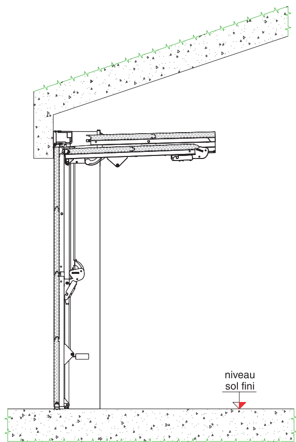
Garage avec plafond en pente
