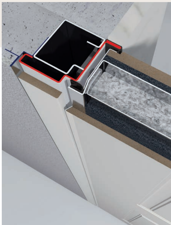
Pose à ras de mur
