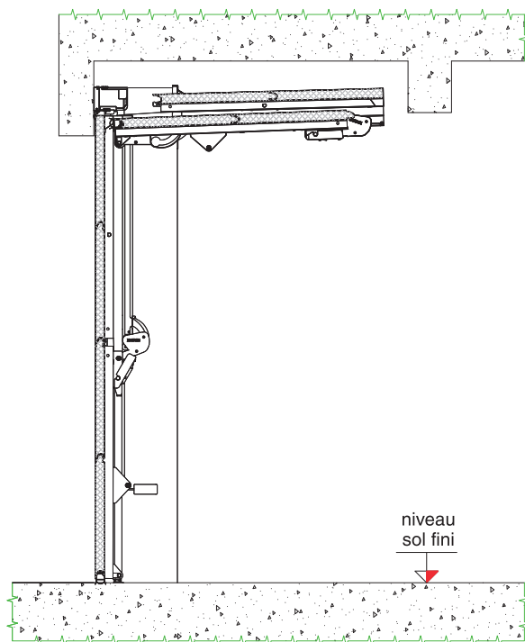
Garage avec linteau
