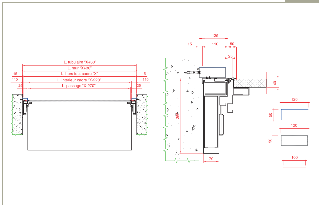
Coupe horizontale - general
